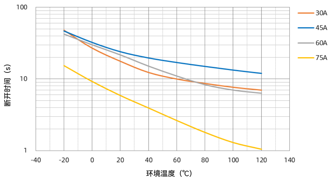
SHP 温度-时间曲线
